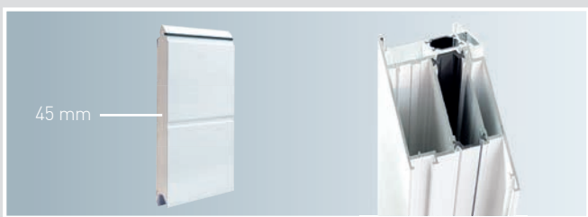
45 mm isolering och termiskt delade profiler (tillval)
